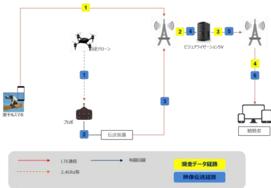
<大会映像配信のシステム構成図>
